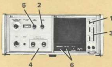
Phase-Magnitude Display—8412A 3
